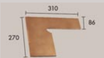
ZANQUÍN VIERTEGUAS
