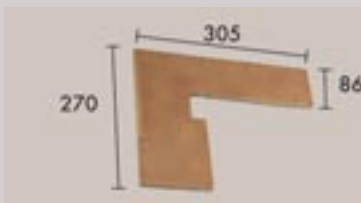
ZANQUÍN RECTO
