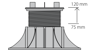
Supporto a testa autolivellante
